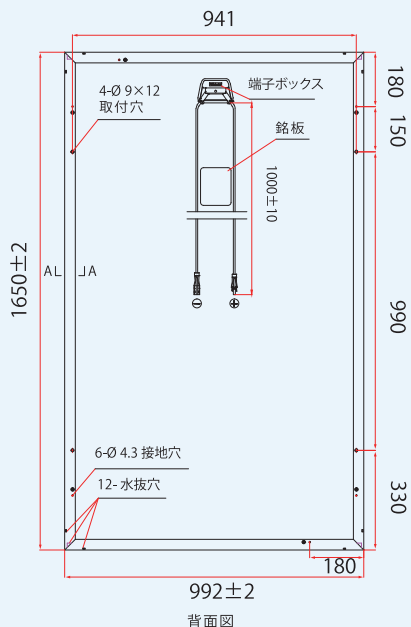
背面図
